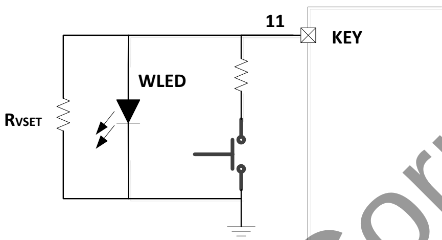
图 7 KEY 按键接法
