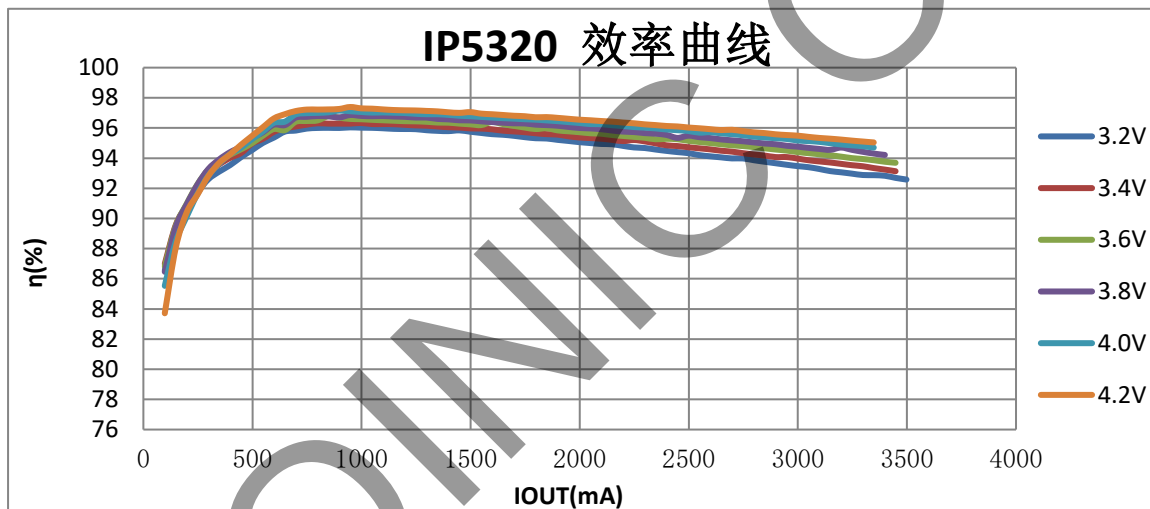
图4 IP5320 效率曲线
