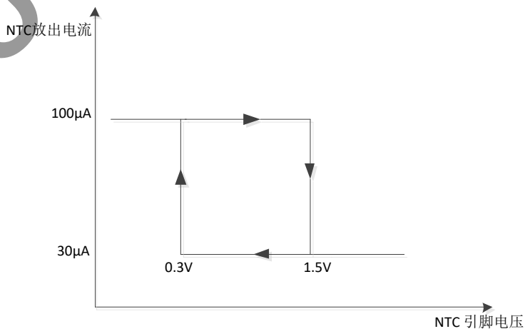
图 12 NTC 电压和放出电流关系
